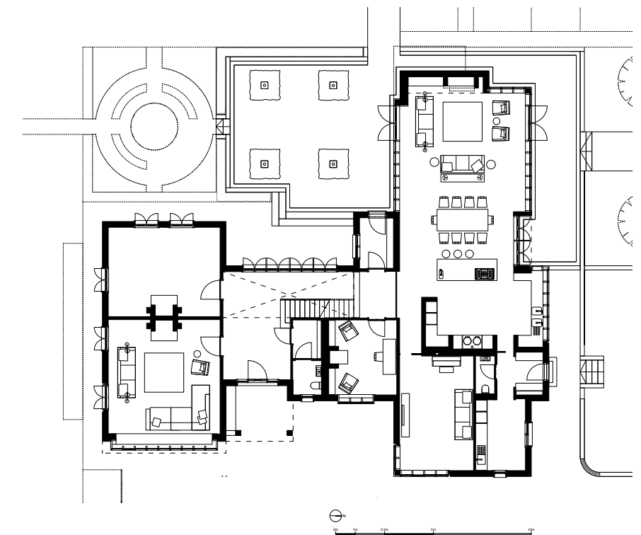
▲ Földszinti alaprajz
